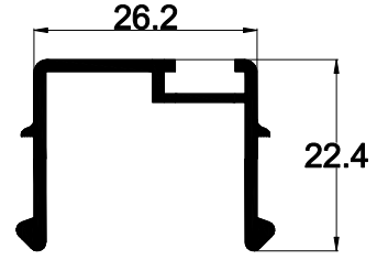
40 E 81 AĞIRLIK : 0.307 kg/mt.
