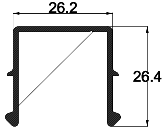
40 E 82 AĞIRLIK : 0.313 kg/mt.
