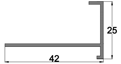
40 E 88 AĞIRLIK : 0.259 kg/mt.
