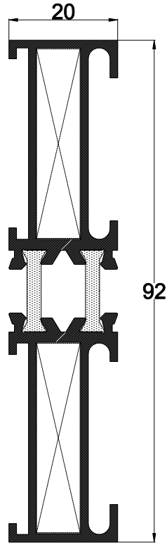
40 E 10 AĞIRLIK : 1.248 kg/mt. JX: 33.56 cm 4 JY: 1.49 cm 4
