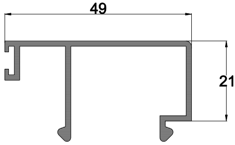
40 E 83 AĞIRLIK : 0.478 kg/mt.
