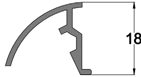
40 E 86 AĞIRLIK : 0.180 kg/mt.
