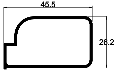
40 E 85 AĞIRLIK : 0.502 kg/mt. JX: 19.67 cm 4 JY: 46.59 cm 4
