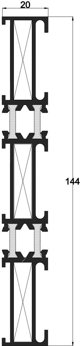
40 E 11 AĞIRLIK : 2.000 kg/mt. JX: 118.77 cm 4 JY: 2.33 cm 4
