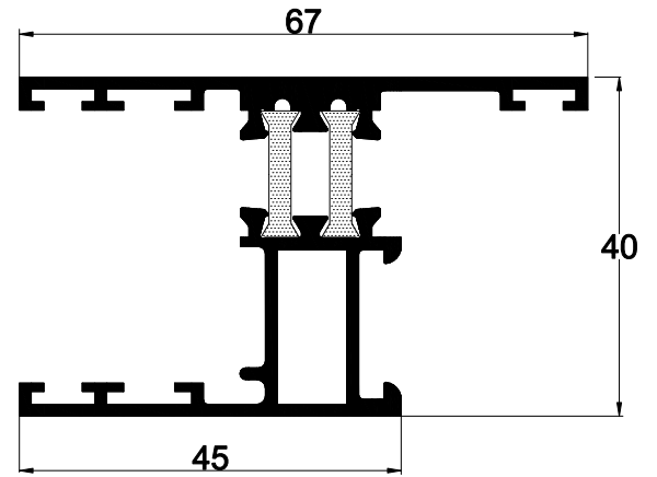
40 E 01 AĞIRLIK : 1.114 kg/mt. JX: 9.37 cm 4 JY: 8.58 cm 4
