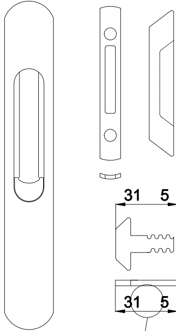
40 D 28 HAVUZLU KİLİT GIESSE BRIO MINI PENCERE İÇİN Ö:1/2
