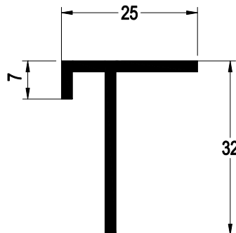
90-259 AĞIRLIK : 0.325 kg/mt.
