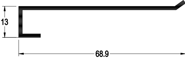
99-1133 AĞIRLIK : 0.358 kg/mt.
