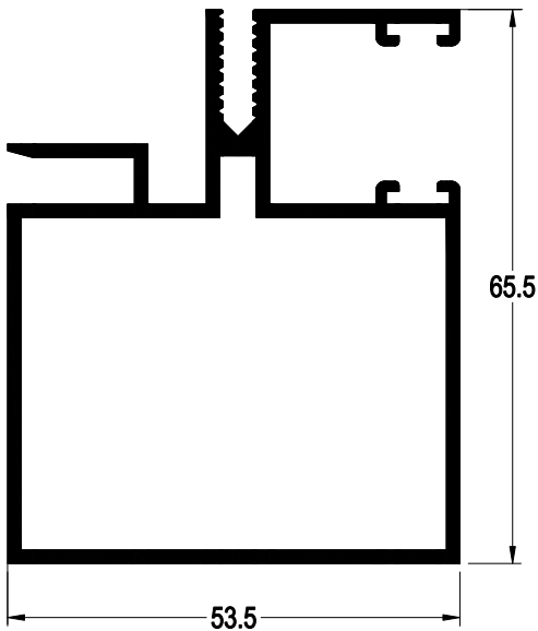
99-1145 AĞIRLIK : 1.282 kg/mt.
