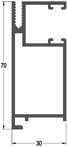
99-1144 AĞIRLIK : 1.037 kg/mt.
