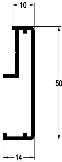
99-1142 AĞIRLIK : 0.409 kg/mt.
