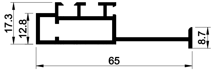
50 E 54 Ağırlık: 0,608 kg/mt
