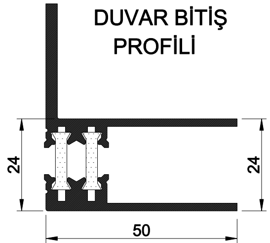
50 E 95 Ağırlık: 1,165 kg/mt
