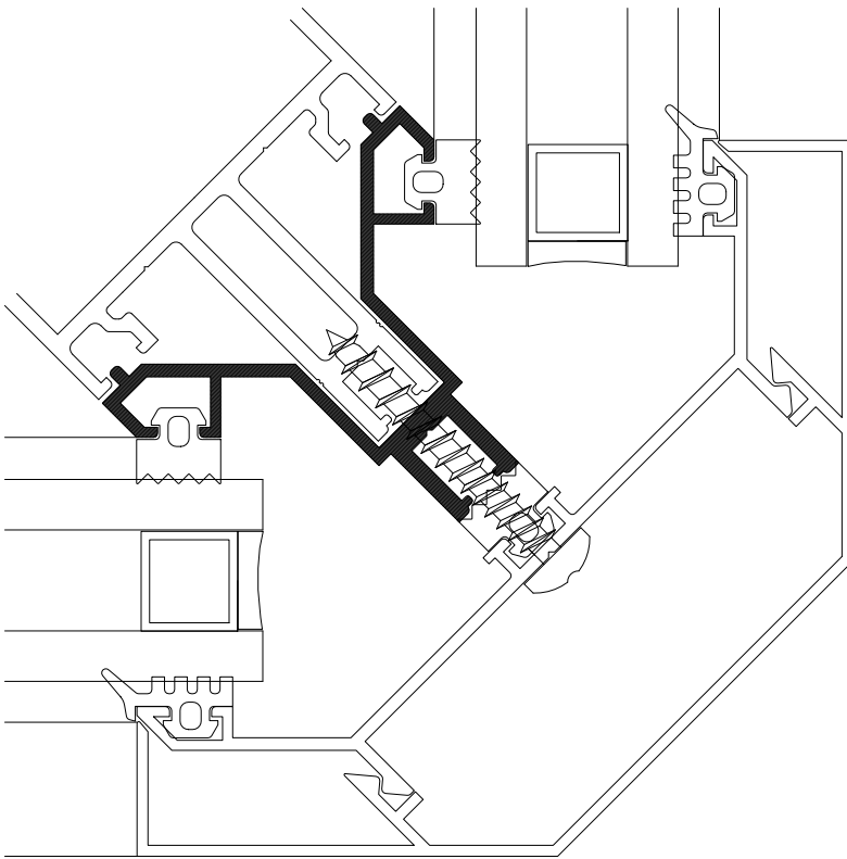
50 E 51 Ağırlık: 0,634 kg/mt
