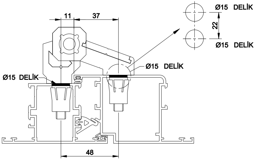
C50 EGZANTRİK MENTEŞE
