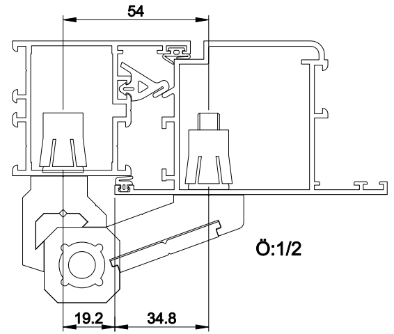
DIŞA AÇILIR KAPI MENTEŞESİ
