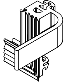
03.06.03.50R KÖŞE FİTİLİ (SAĞ) CORNER GASKET (RIGHT) EPDM 01.02.03.50R - 01.03.03.50R
