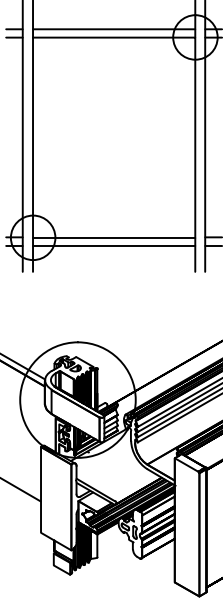
03.05.03.50R KÖŞE FİTİLİ (SOL) CORNER GASKET (LEFT) EPDM 01.02.03.50R - 01.03.03.50R
