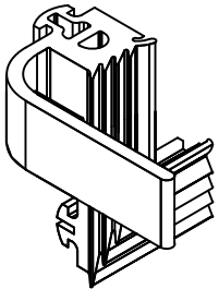
03.05.07.50R KÖŞE FİTİLİ (SOL) CORNER GASKET (LEFT) EPDM 01.02.07.50R - 01.03.07.50R
