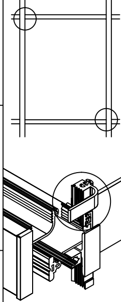
03.06.03.50R KÖŞE FİTİLİ (SAĞ) CORNER GASKET (RIGHT) EPDM 01.02.03.50R - 01.03.03.50R
