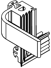
03.05.04.50R KÖŞE FİTİLİ (SOL) CORNER GASKET (LEFT) EPDM 01.02.04.50R - 01.03.04.50R
