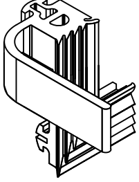
03.05.02.50R KÖŞE FİTİLİ (SOL) CORNER GASKET (LEFT) EPDM 01.02.02.50R - 01.03.02.50R
