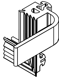
03.06.07.50R KÖŞE FİTİLİ (SAĞ) CORNER GASKET (RIGHT) EPDM 01.02.07.50R - 01.03.07.50R
