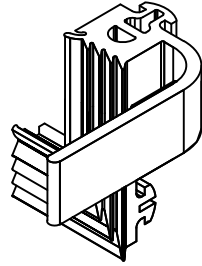
03.06.04.50R KÖŞE FİTİLİ (SAĞ) CORNER GASKET (RIGHT) EPDM 01.02.04.50R - 01.03.04.50R
